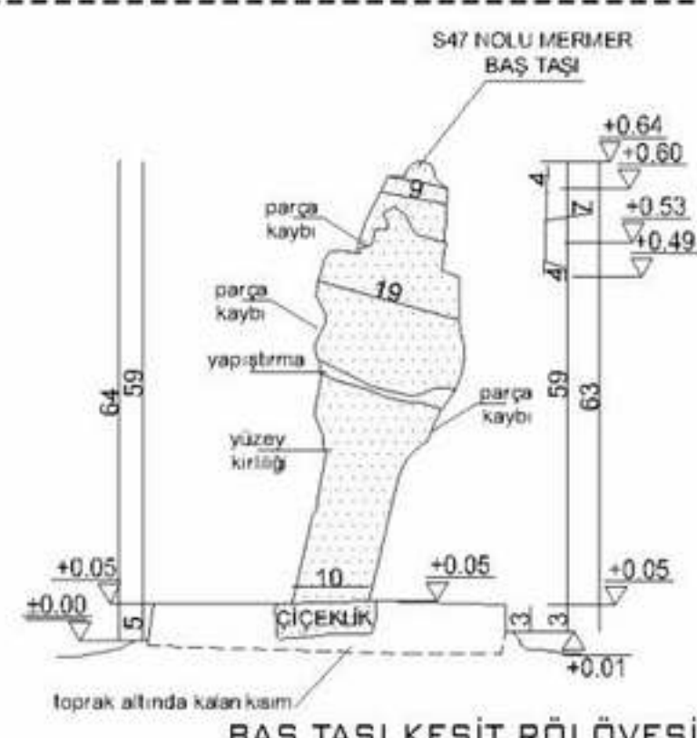
BAŞ TAŞI KESİT RÖLÖVESİ
