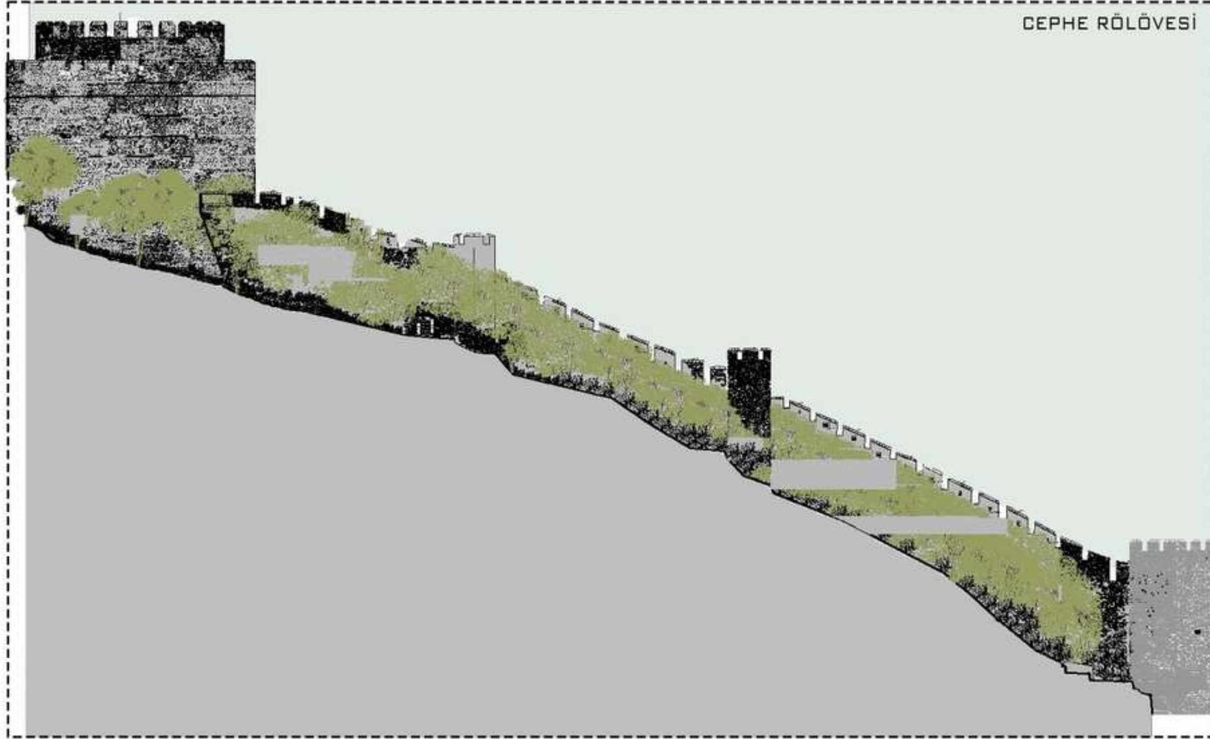
BOĞAZ CEPHE RÖLÖVESİ
