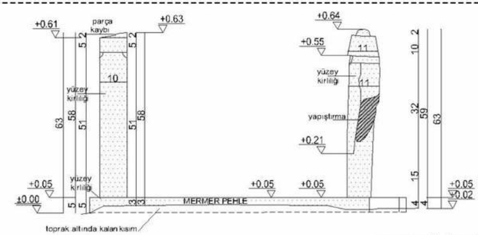
CEPHE RÖLÖVESİ
