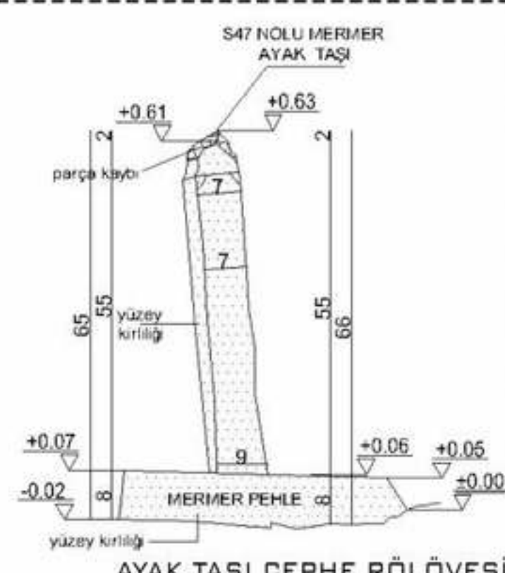
AYAK TAŞI CEPHE RÖLÖVESİ
