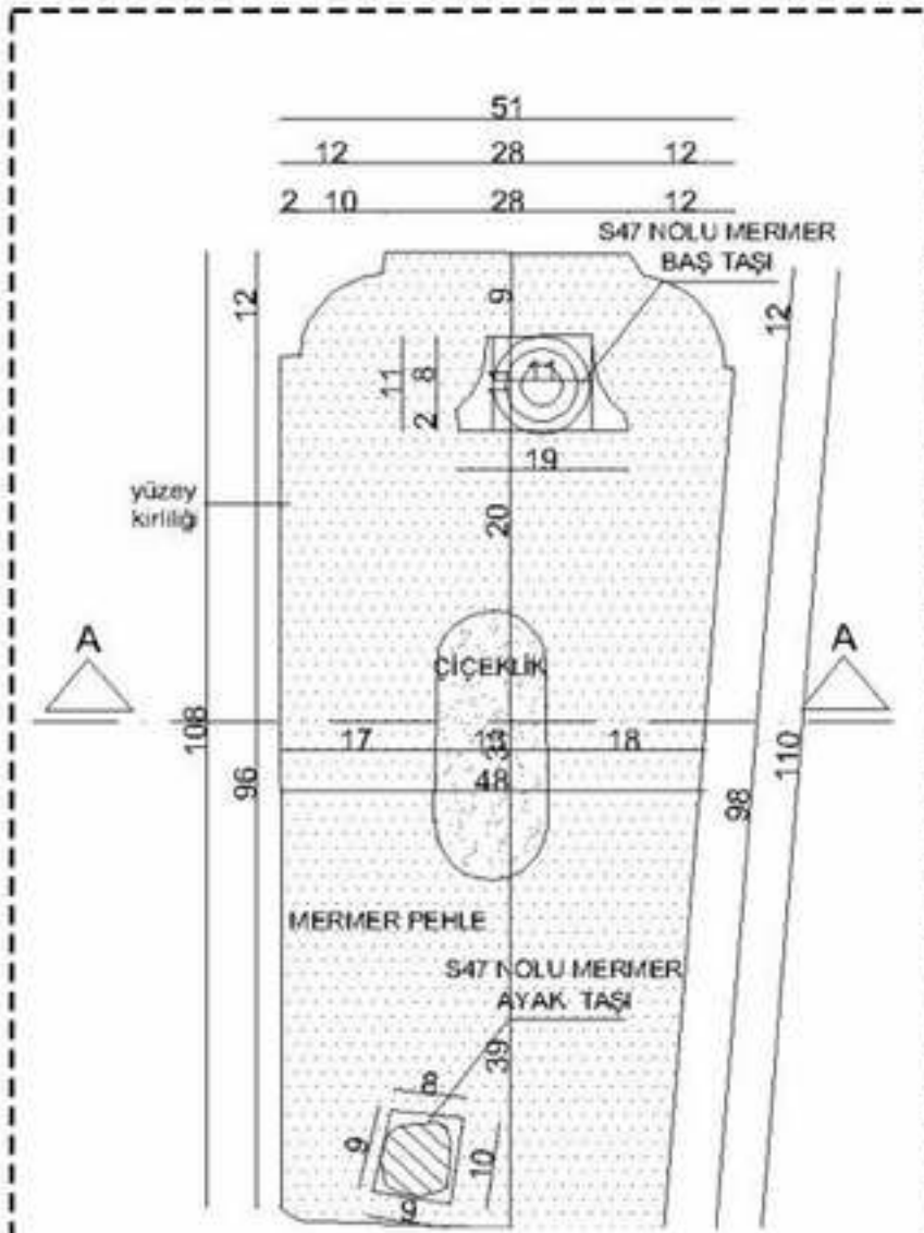
PLAN RÖLÖVESİ
