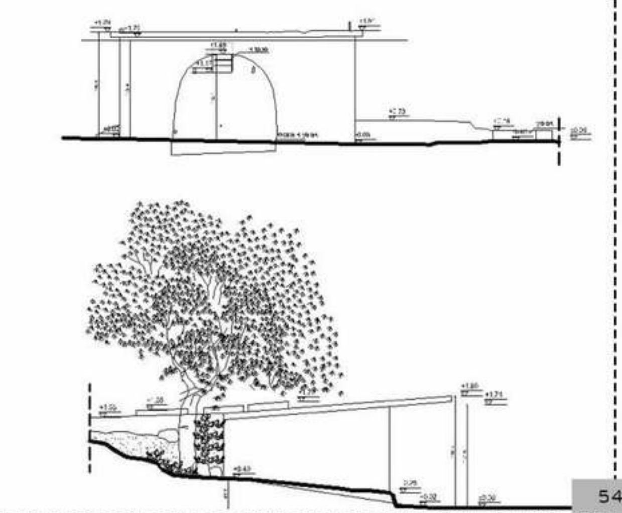
CEPHE RÖLÖVESİ
