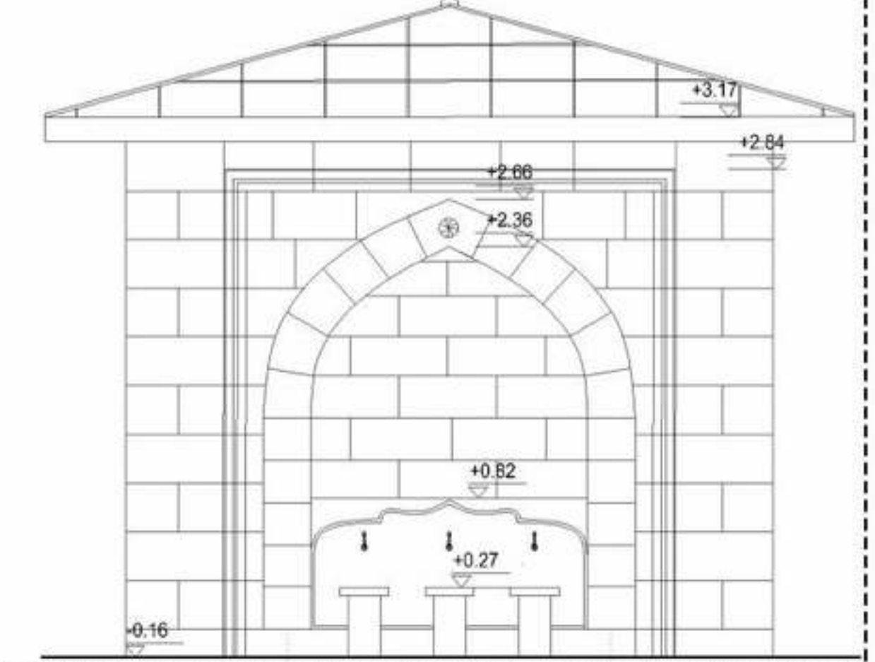
CEPHE REKONSTRÜKSİYONU
