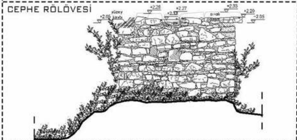
CEPHE RÖLÖVESİ
