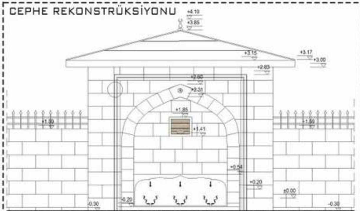
CEPHE REKONSTRÜKSİYONU
