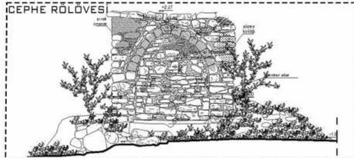
CEPHE RÖLÖVESİ
